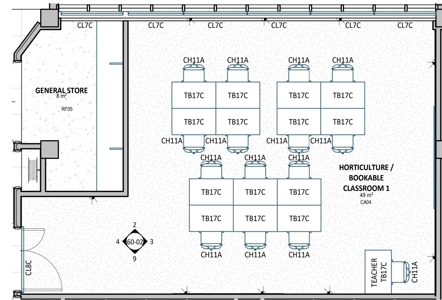
1 PLAN DETAIL 1 : 50
