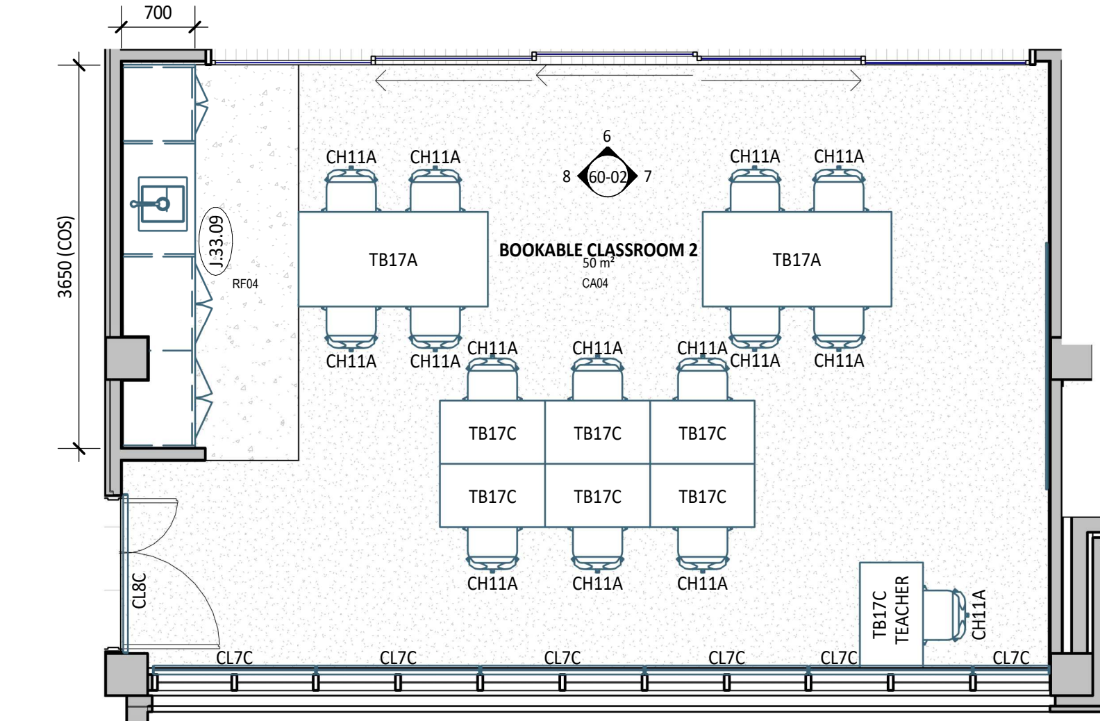
5 PLAN DETAIL 1 : 50
